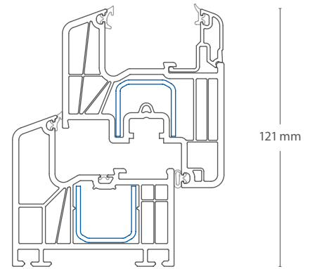
Anschlagdichtung (AD) Abb.: 1:2,5
