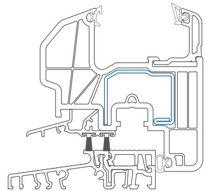
Flache Aluminium Bodenschwelle: Höhe 20 mm Abb.: 1:2
