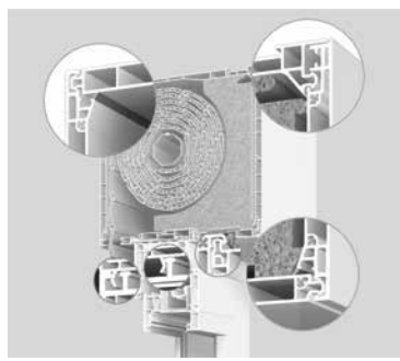
Dichtungen zwischen den Profilen für höchste Luftdichtheit
