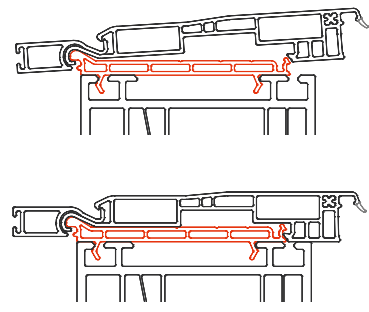
Schnelles und einfaches Aufklipsen des Kastens auf das Fenster.
